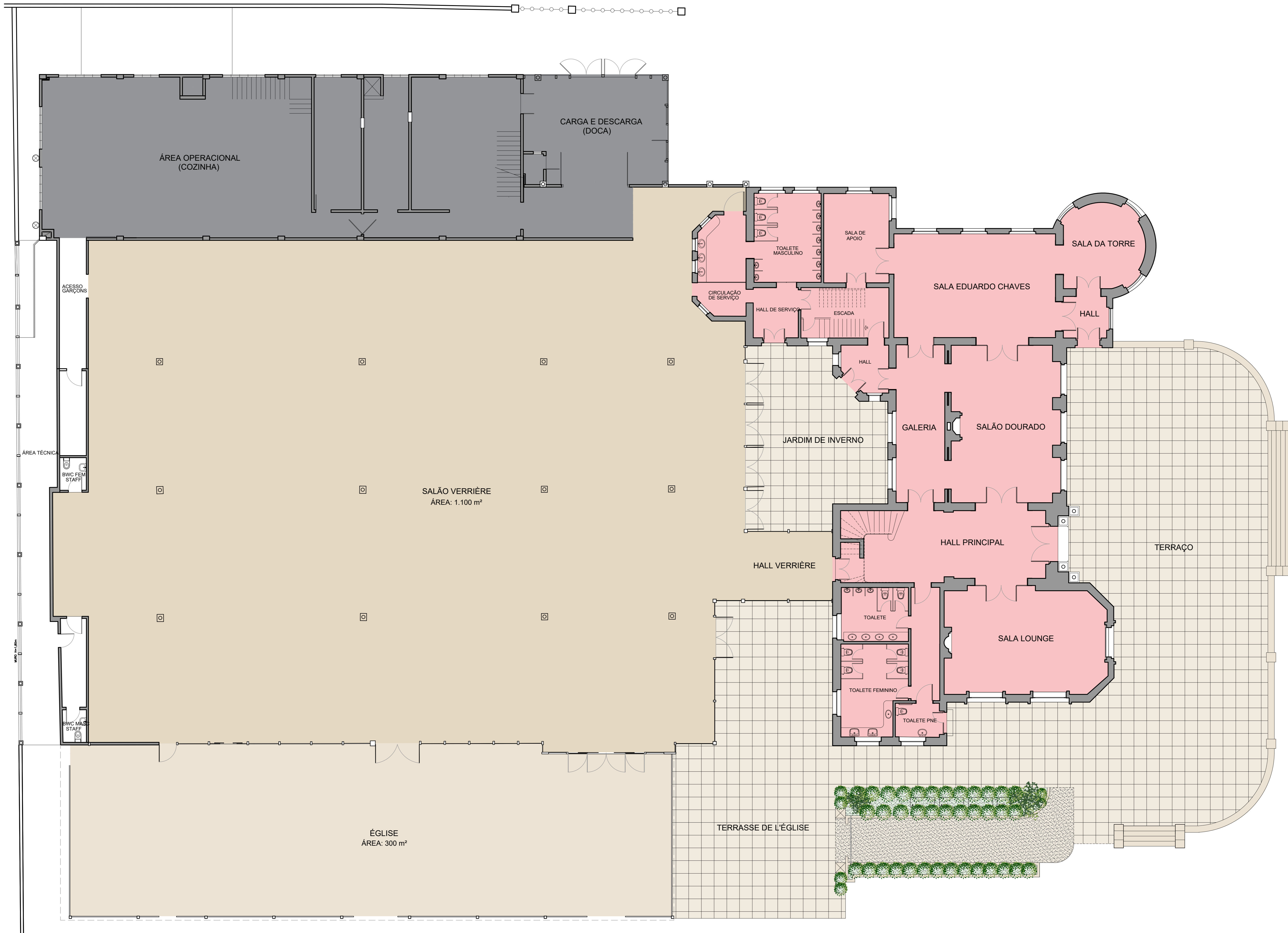
PLANTA - CASTELO DO BATEL ESCALA 1/100
